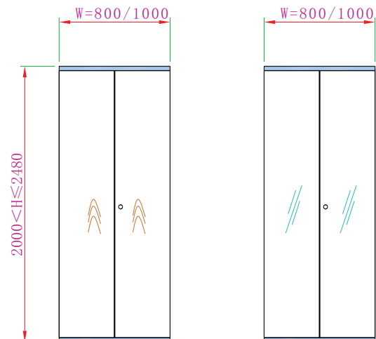
功能柜（CUQG01） -单/双开木门
