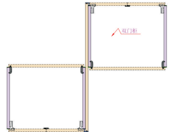
Z连接
