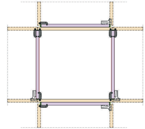
十字连接
