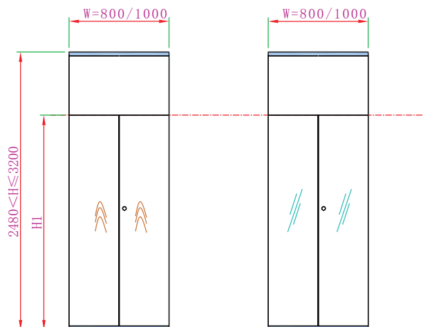
功能柜 (CUQG02) -双开木门
