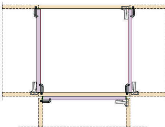
T连接
