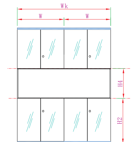
大空格柜（CUQG24）-双开玻璃门
