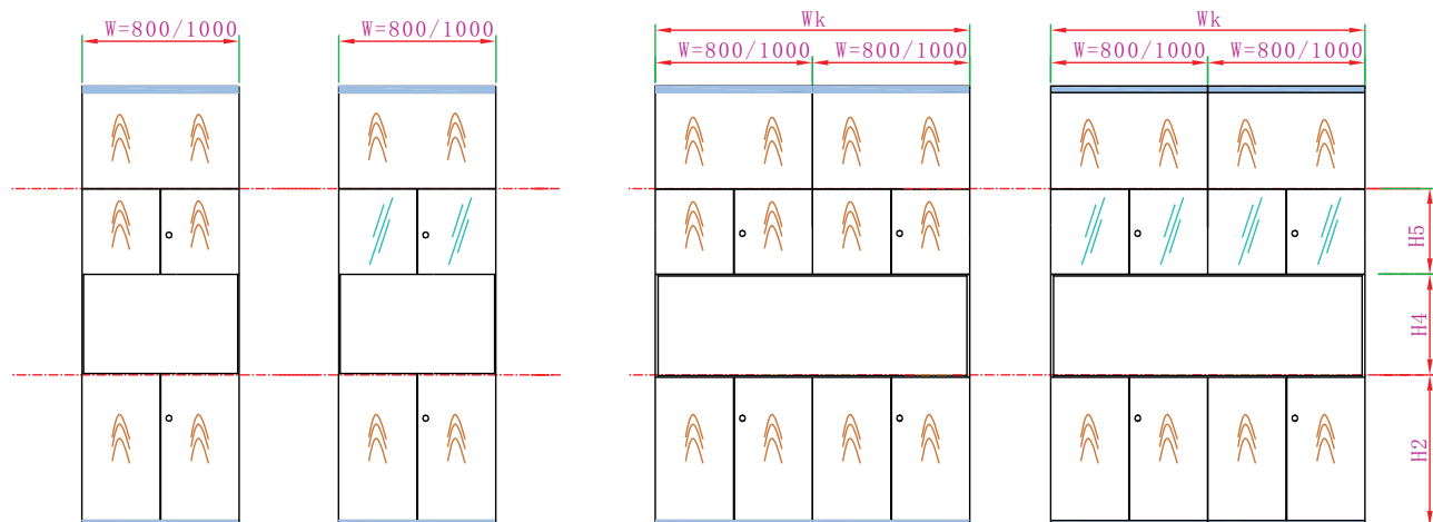
小空格柜(CUQG22) -单开木门
