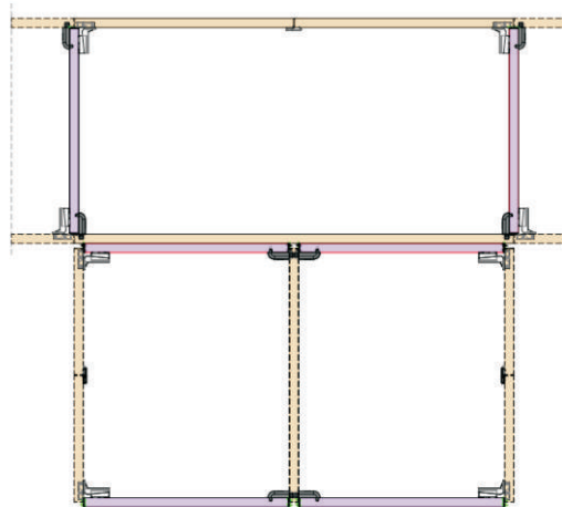
双背板柜T连接
