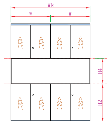
大空格柜（CUQG24）-双开木门
