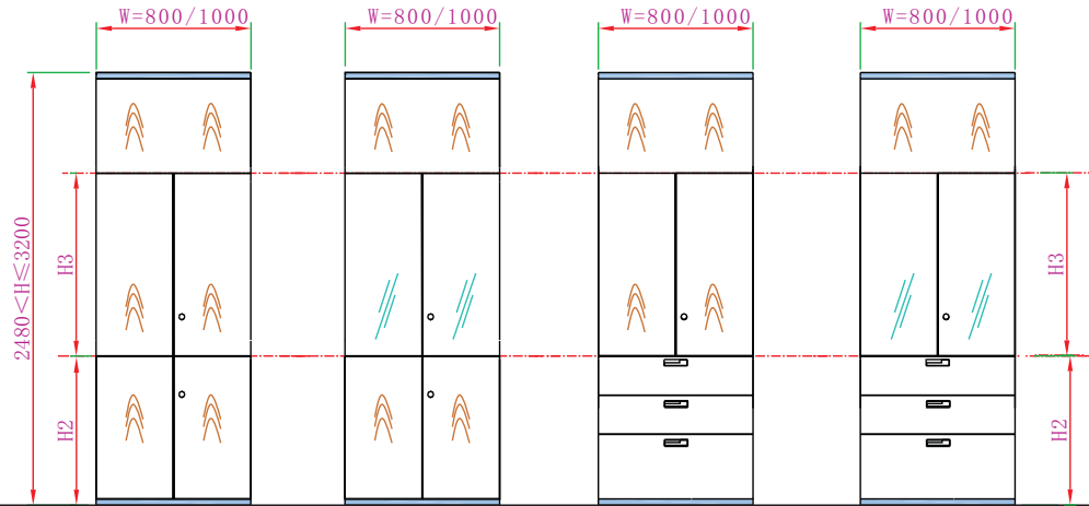
层板柜(CUQG13) -双开木门
